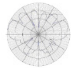
OD49M-6 E-Plane
