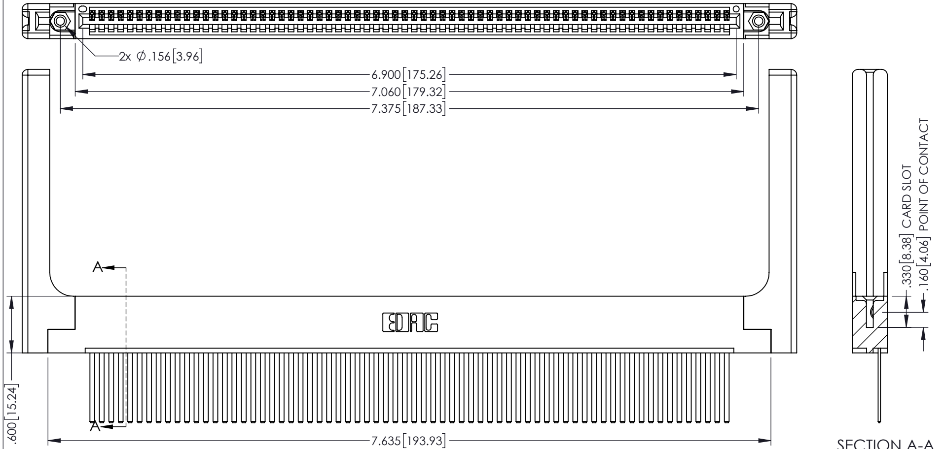
SECTION A-A
