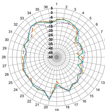
YZ-Plane Gain
