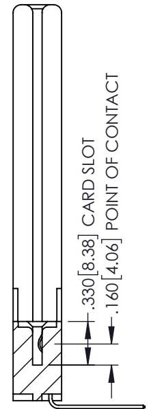
SECTION A-A
