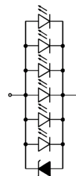
【 Inside circuit 】
