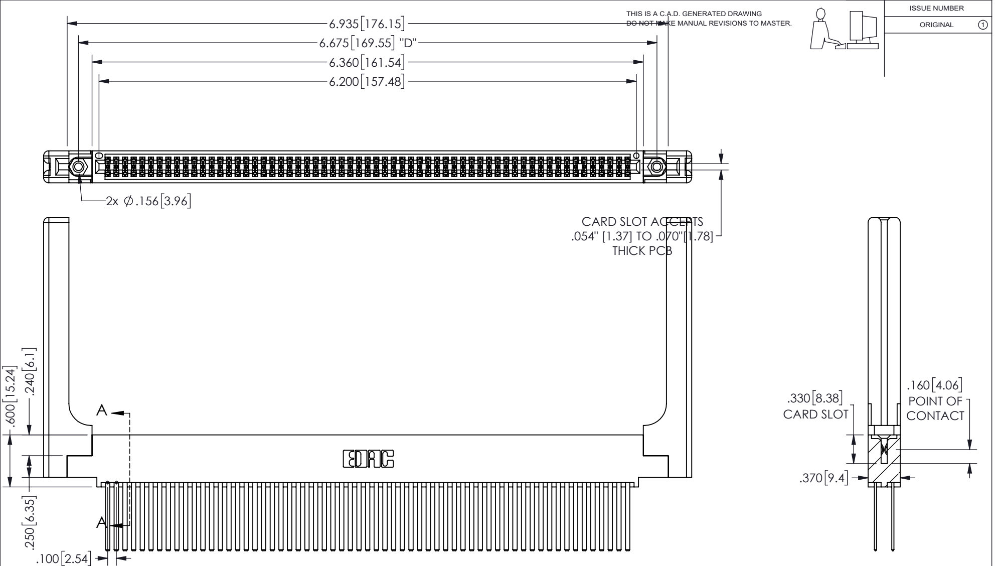
SECTION A-A
