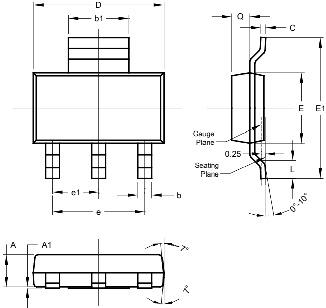
SOT223
