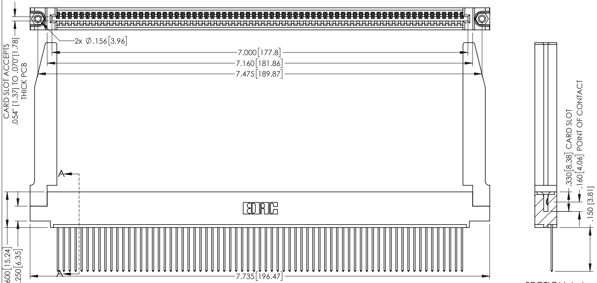
SECTION A-A
