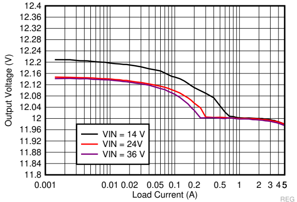
V_{OUT} = 12\text{ V} f_{SW} = 500\text{ kHz} Auto Mode
