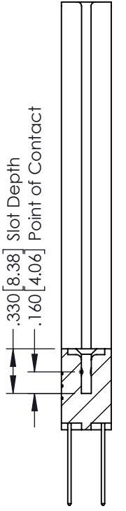
SECTION A-A
