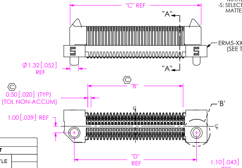
FIG 1 ERM5-030-02.0-X-DV-XX SHOWN
