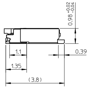
ACTUATOR CLOSE
