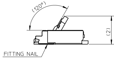
ACTUATOR OPEN
