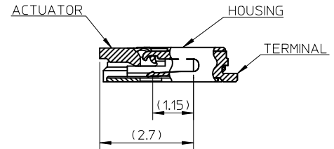
SECTION V-V SCALE 15:1
