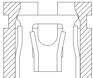
A-A Section
