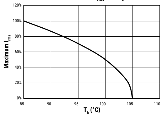
Maximum I_{rms} vs. T_h
