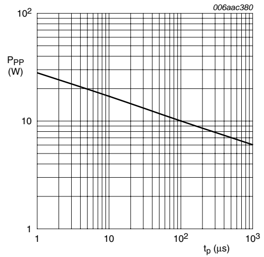
T_{amb} = 25\text{ °C} (1) PESD9V0V4UK
