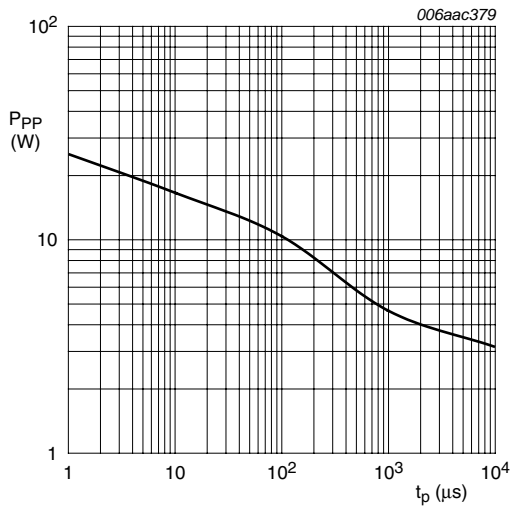
T_{amb} = 25\text{ °C} (1) PESD3V3V4UK (2) PESD5V0V4UK
