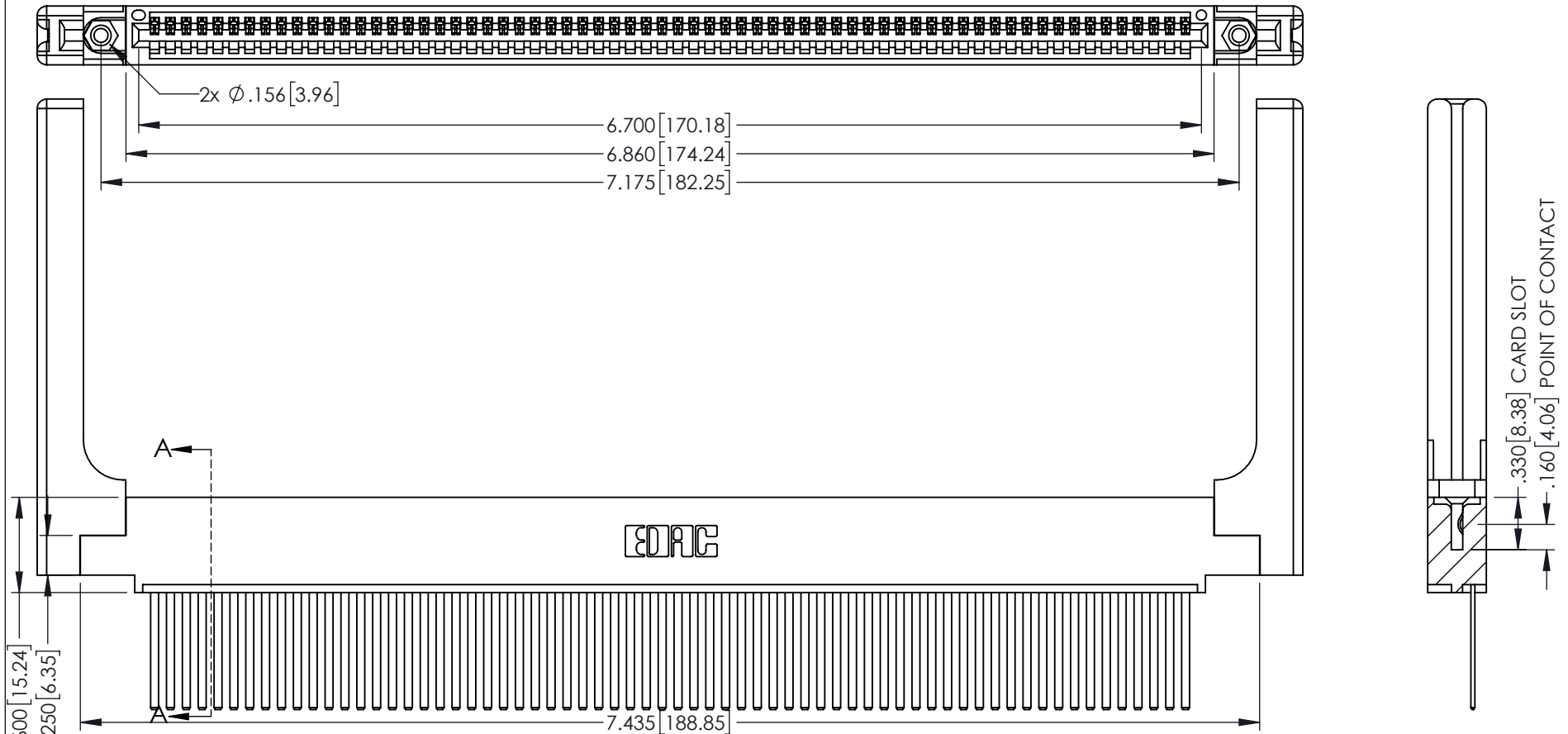
SECTION A-A
