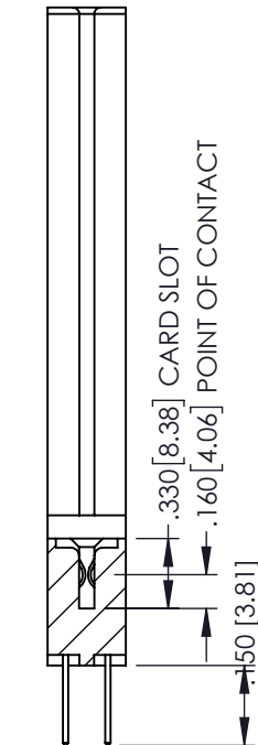
SECTION A-A
