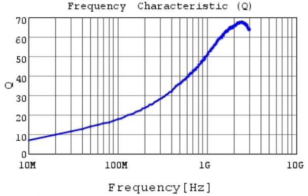
LQG15WH4N1S02 Q
