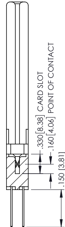
SECTION A-A
