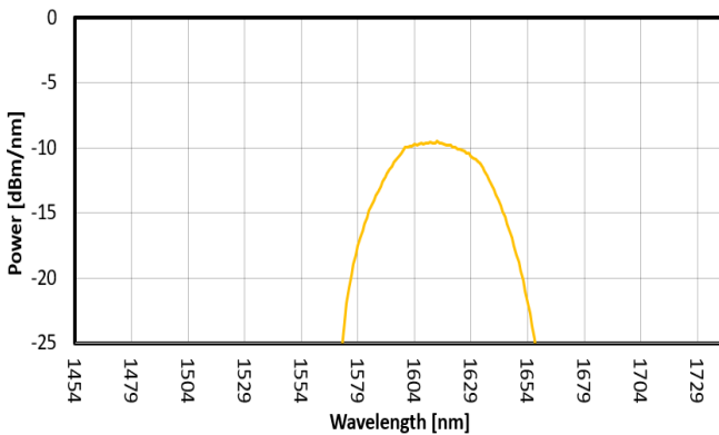
FIG. 3: SLED 2 SPECTRUM
