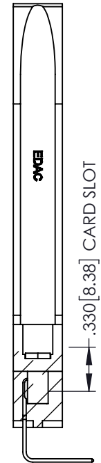
SECTION A-A
