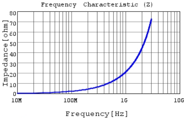
LQG15WZ3N4S02 |Z|
