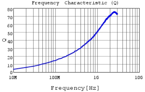
LQG15WZ3N4S02 Q
