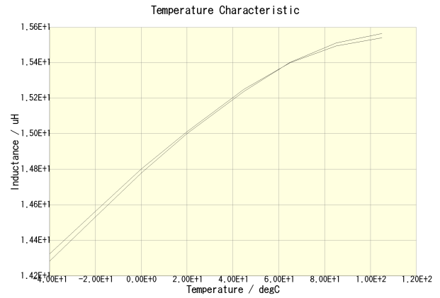
CLF12555T-150M-CA(DC = 0A)
