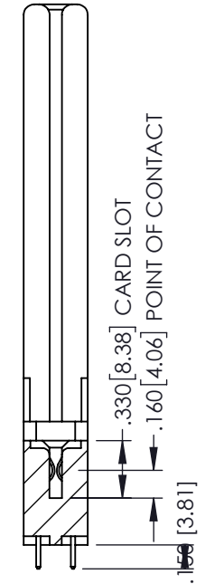
SECTION A-A
