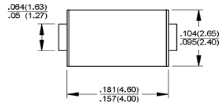
DO-214AC (SMA)
