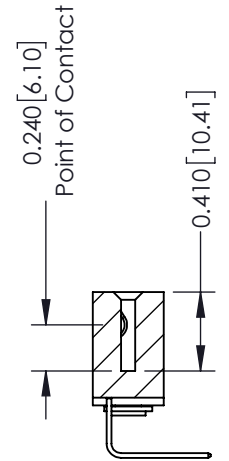
SECTION A-A
