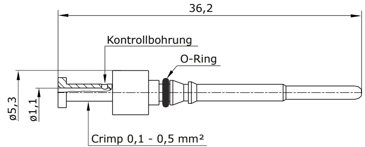
Hauptabmessungen Kontaktstift
