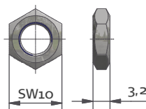
Mutter | nut M6 x 0,35
