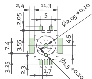
Löt-Pad-Anordnung SMD soldering pad
