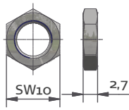
Mutter | nut M7 x 0,75
