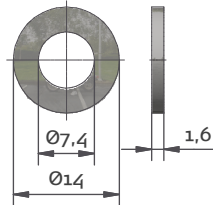
Scheibe | washer DIN 125
