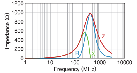
MMZ1608D241CTD25
