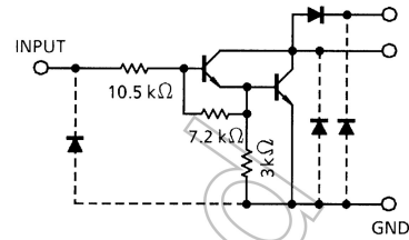
ULN2804APG / AFWG
