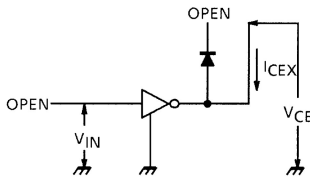
1. I_{CEX}
