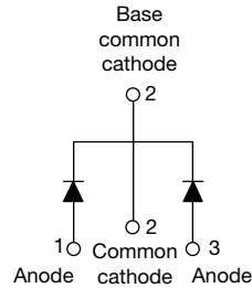
VS-40CTQ150-1HM3
