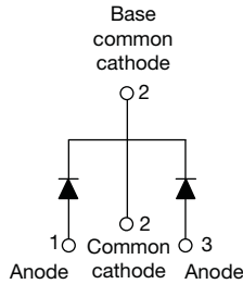
VS-40CTQ150SHM3
