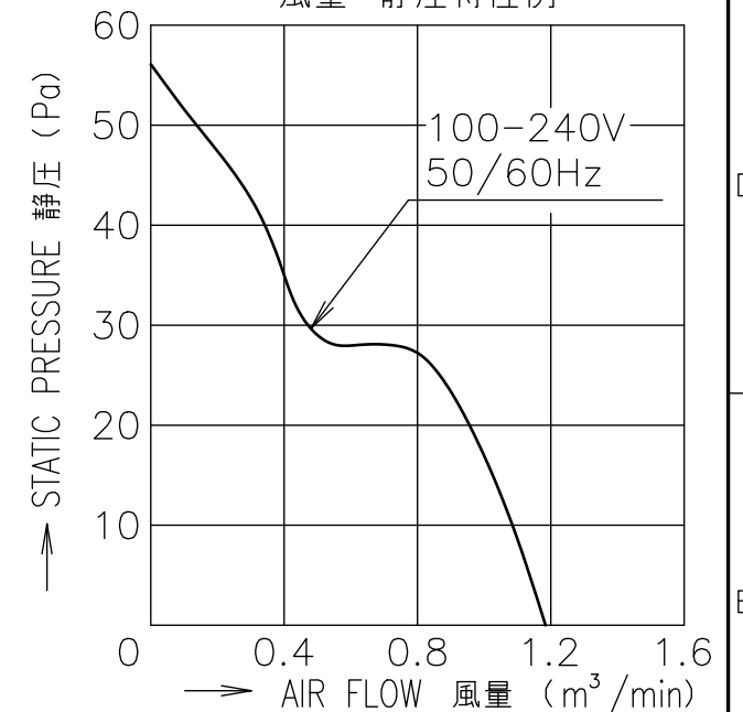
風量-静圧特性例
