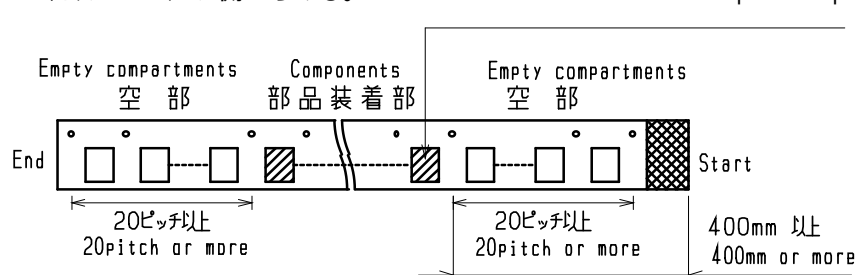
上面図 (Top view)
