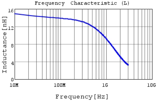
LQW18CN15NJ0Z L
