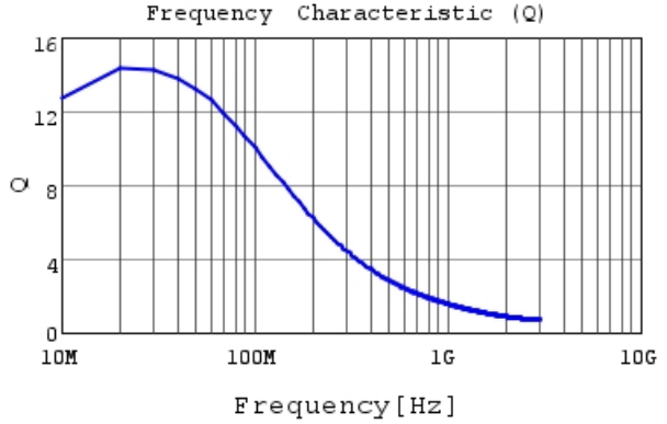
LQW18CN15NJ0Z Q
