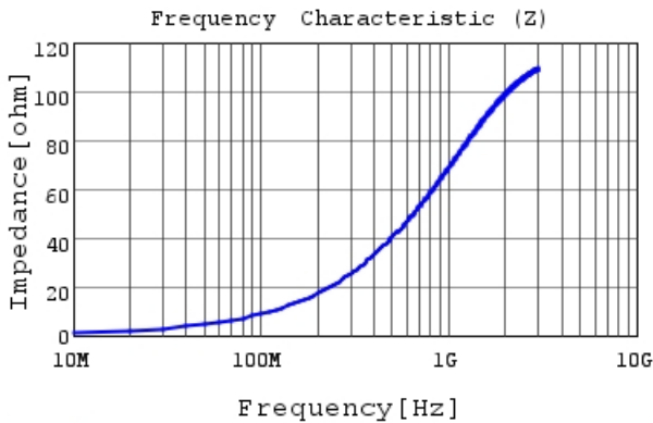
LQW18CN15NJ0Z |Z|
