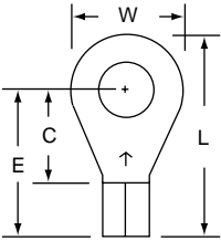
MU10-14R/S Stud Size 1/4 Wire Range 12-10
