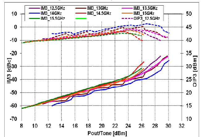
@Vds=6V, Ids=2500mA
