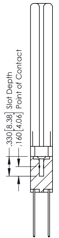
SECTION A-A
