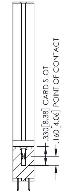
SECTION A-A
