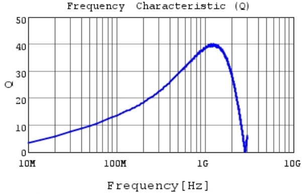
LQG15WZ22NH02 Q
