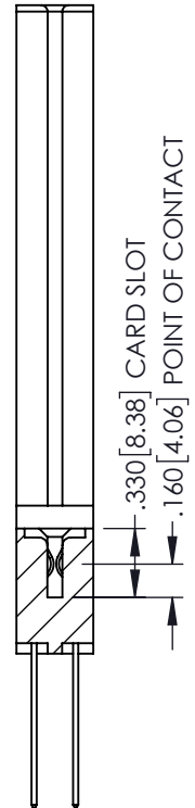
SECTION A-A
