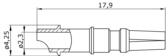
Hauptabmessungen Kontaktbuchse
