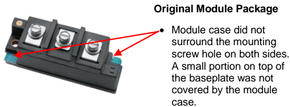
Original Module Package
