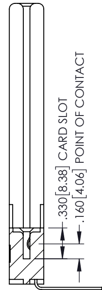
SECTION A-A
