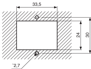
99 766 6 : Panel cut-out
