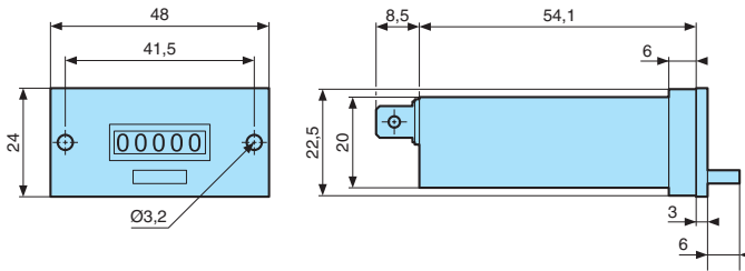
99 766 92 : 24 x 48 - 5 decades
