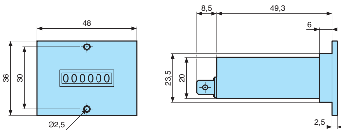
99 766 70 : 36 x 48 : 6 decades
