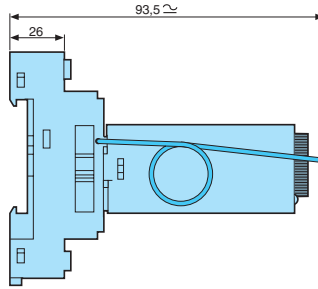
PCB base RTMA4 - 26 532 708
