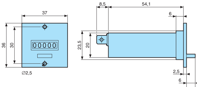
99 766 61 : 36 x 37 - 5 decades
