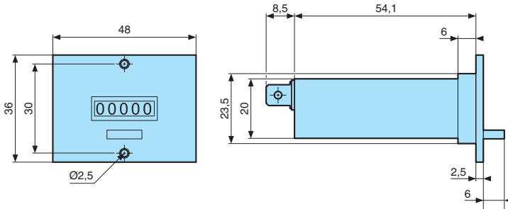
99 766 71 : 36 x 48 - 5 decades
