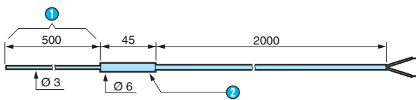
Thermocouple probe K : 79 696 034
