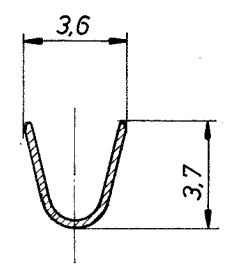
Schnitt: C - C
