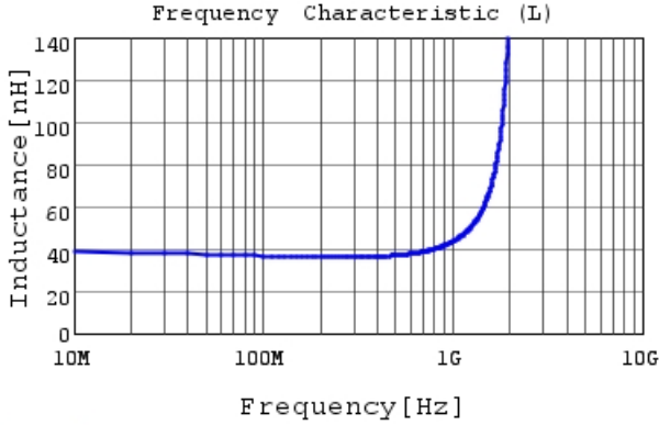
LQG15WH36NG02 L
