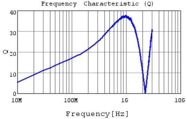
LQG15WH36NG02 Q
