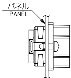
パネル前面取り付け FRONT MOUNT TYPE
